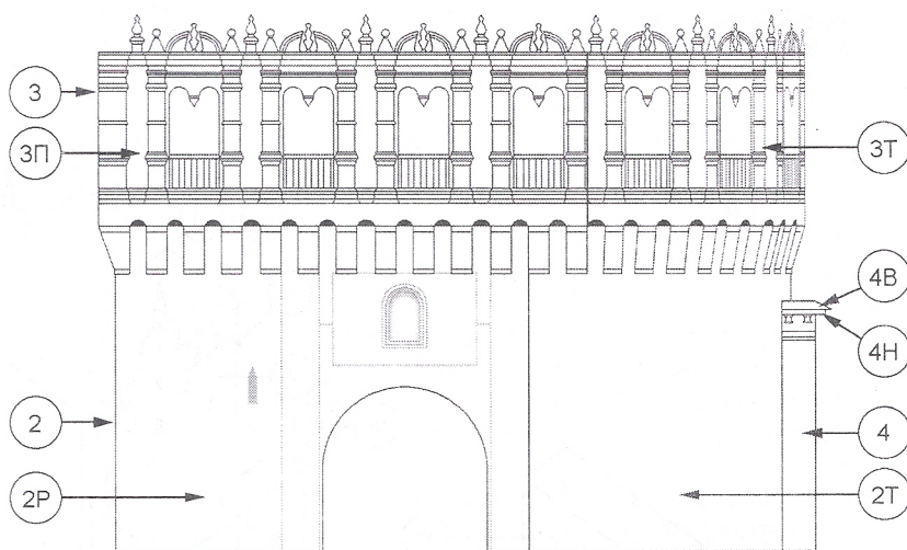
ПОСЛЕДОВАТЕЛЬНОСТЬ СБОРКИ МОДЕЛИ БАШНИ
