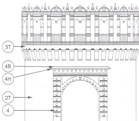
ПОСЛЕДОВАТЕЛЬНОСТЬ СБОРКИ МОДЕЛИ БАШНИ
